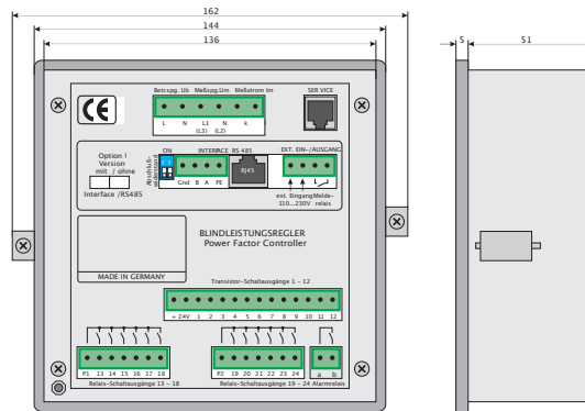
Maßbild PFC-12TR-1/PFC-12TR-1-RS485
