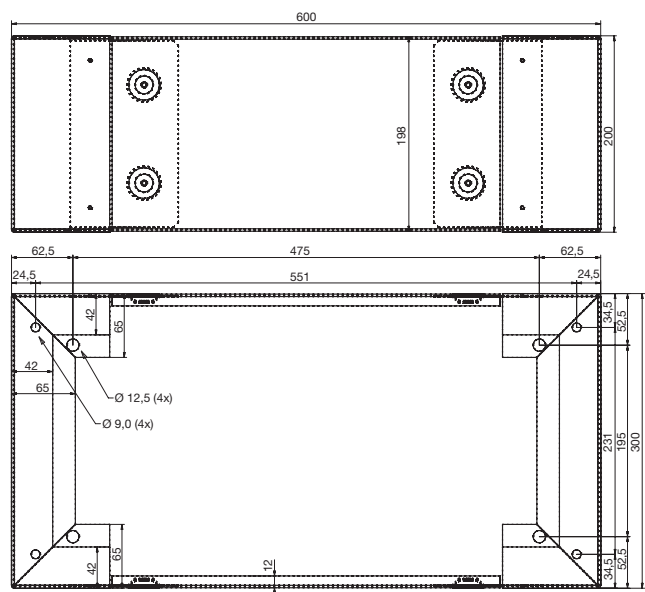
Maßbild Socket LSK-3
