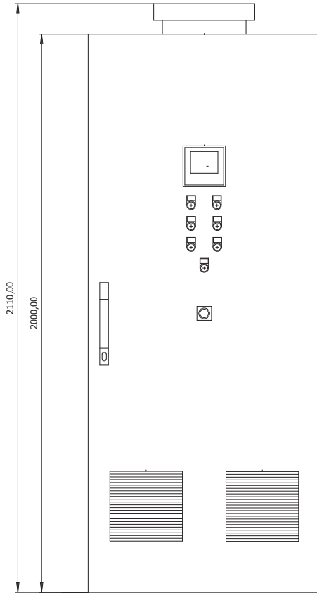
Frontansicht aussen
