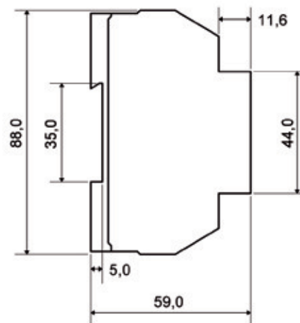
Maßbild EMB 1101
