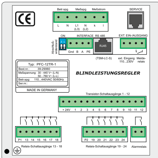
Bild 2: Rückansicht
