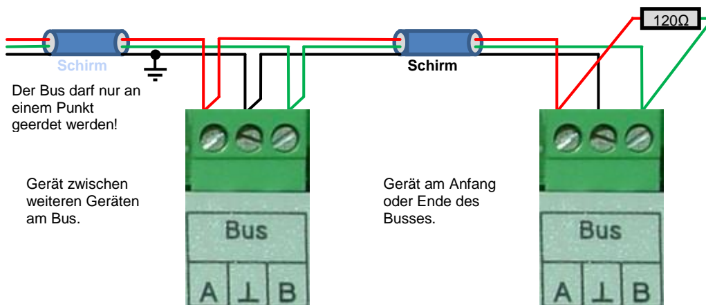
Abbildung 7: FRAKO-Starkstrombus
